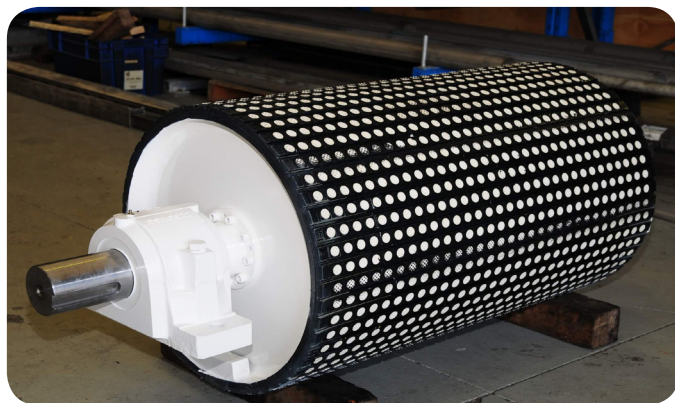
Ceramic Lagging
